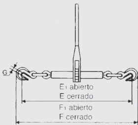
MODELO PTG Tensor de carraca con ganchos
